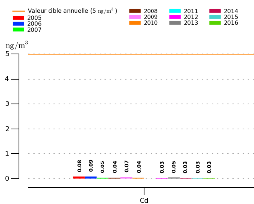
Illustration 38: Evolution annuelle des concentrations de cadmium en air ambiant
